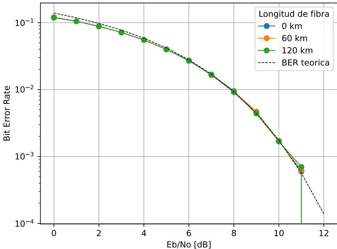
BER con Modelo de Fibra. Mod: QAM-16. BR = 120 GBd.
